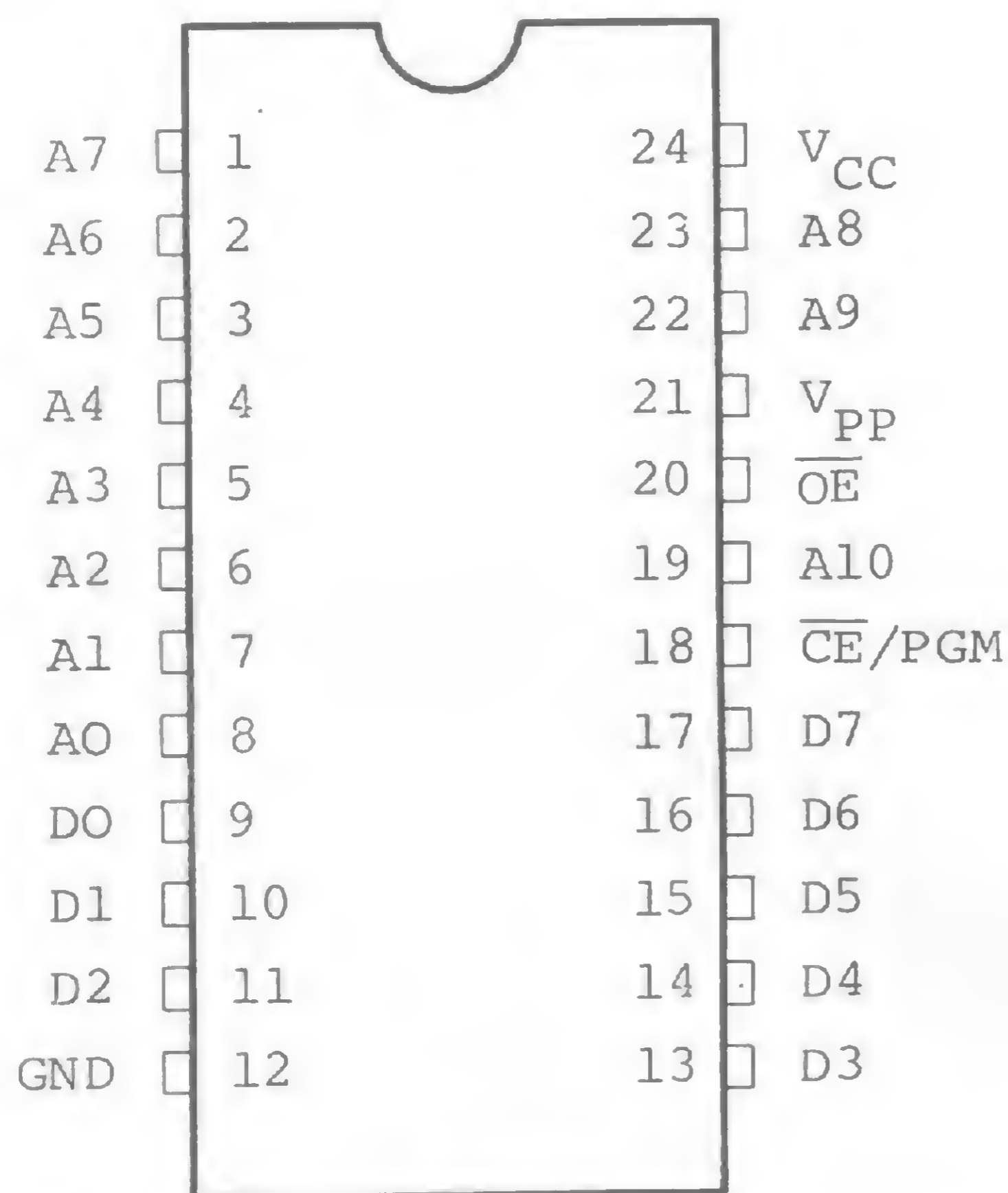
Figura A – Pinagem da EPROM 2716
